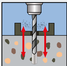
2. Poista pöly
