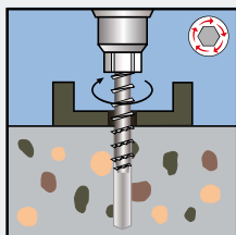
3. Asenna*
