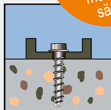
4. Valmis
